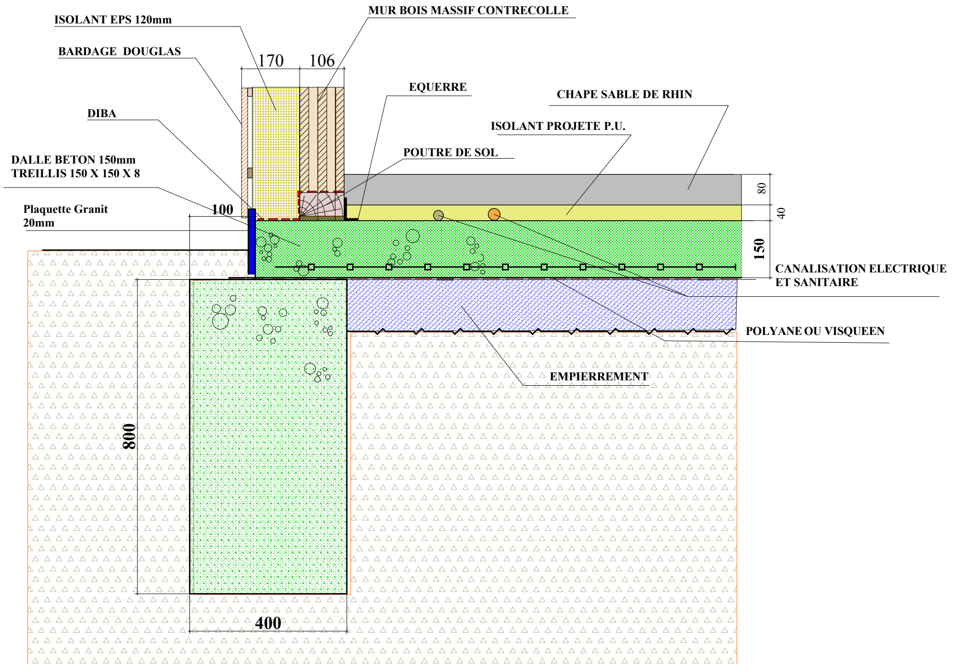
POUTRE DE CEINTURE ET DALLE
